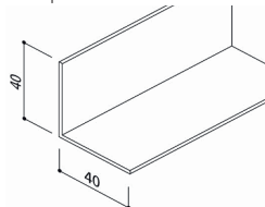
Art. nr. 6087 hoekprofiel 40x40x2
