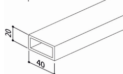
Art. nr. 12740 kokerprofiel 40x20x3
