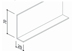
Art. nr. 6023 hoekprofiel 20x70x2
