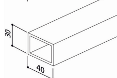
Art. nr. 12741 kokerprofiel 40x30x3
