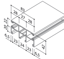
Art. nr. 3060 BB-LHTF
