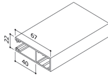
Art. nr. 3045 B-LHTF 120
