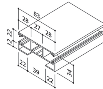
Art. nr. 3047 B-LHTF 150
