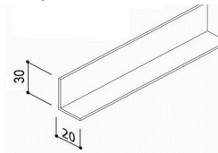
Art. nr. 6022 hoekprofiel 20x30x2
